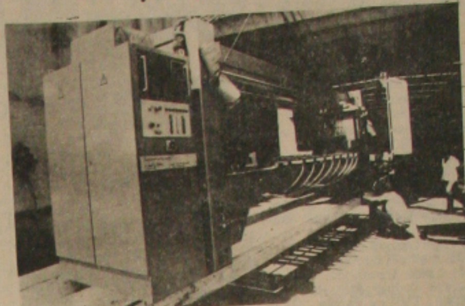
A furadeira automática computadorizada, importada da Alemanha, realiza operações individualizadas, em sequência, autoreajustando-se.
