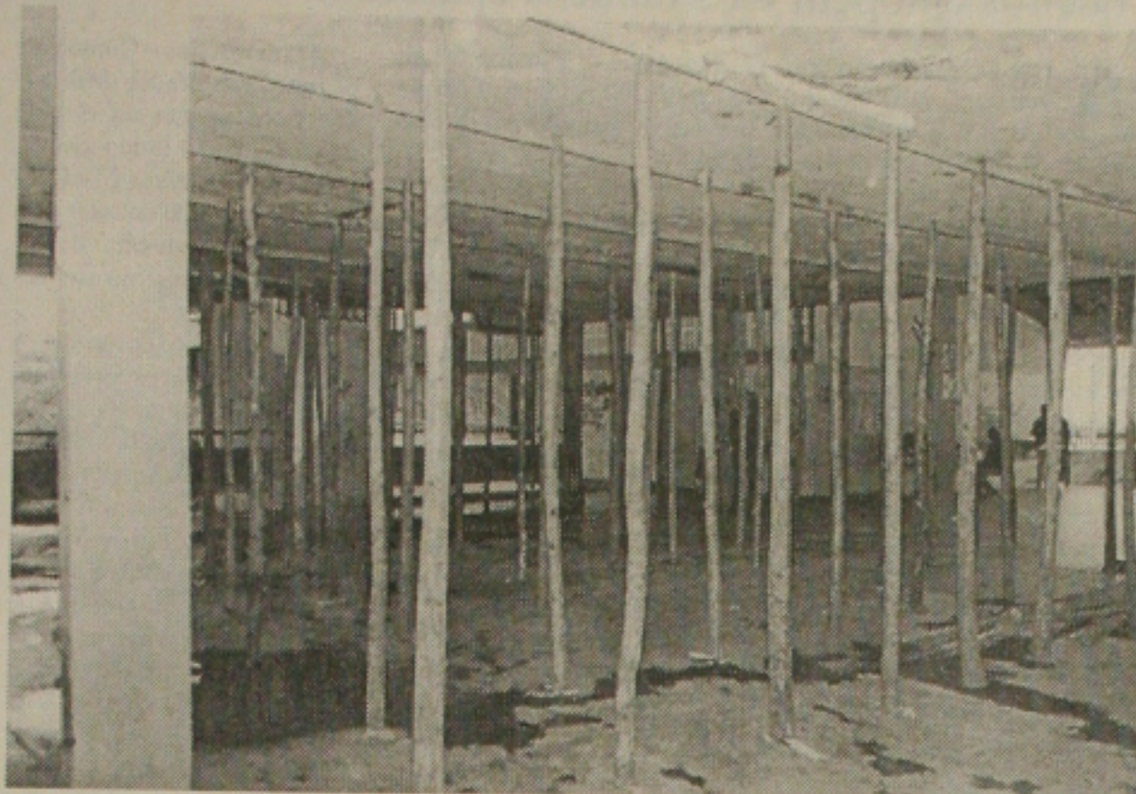
Vigas que sustentam laje do primeiro piso do colégio João Alves Filho
