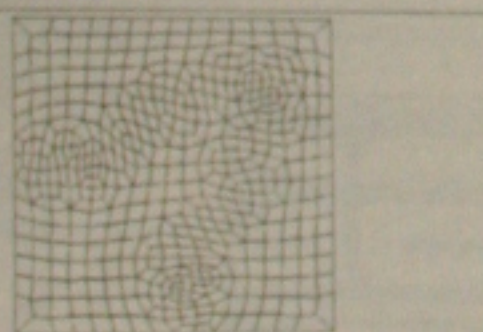
Figura 1. Geração de malha adaptativa quadrilateral típica de fluxo de petróleo.
