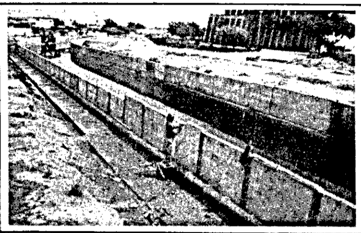
Revestimento do canal da Avenida Gonçalves Prado.
