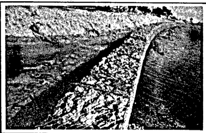
Gabiões de contenção no cais da Marinha da Coroa do Meio.
