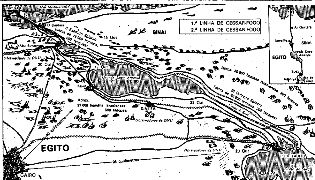
Este é o mapa da situação da Guerra do Oriente Médio, na frente do Sinai, destacando-se as linhas do 1.º e 2.º cessar fogo.
