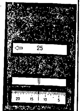
360° Limbo horizontal división sinistrorsum 25° 12' 30"
