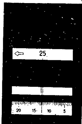
360° Limbo horizontal división sinistrorsum 25° 12' 30"
