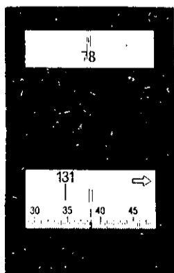
360° Límbo vertical 78° 48' 30"
