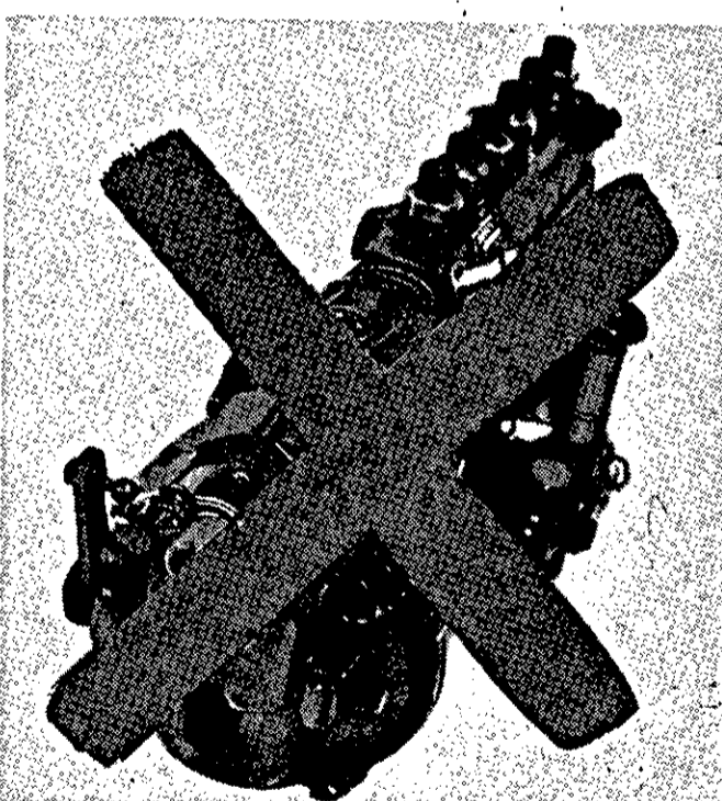
Bomba injetora desregulada. Potência: maior em 8%. Consumo de combustível: maior em 30%.
