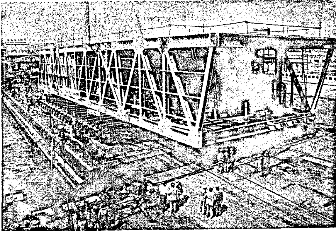
Uma central de energia de uma só peça, com 1.700 toneladas montadas sobre 640 rodas de bôgui - provavelmente a maior carga já transportada por pneumáticos -, é içada para uma barcaça para a primeira fase de sua viagem de Walsend, nordeste da Inglaterra, para o campo de Calymore, no Mar do Norte.
