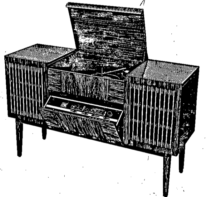
Radiofone FM estéreo Philips RF 646 Amplificador de 20 W, rádio FM estéreo e mais 3 faixas de onda. Toca-discos com cambiador automático.
