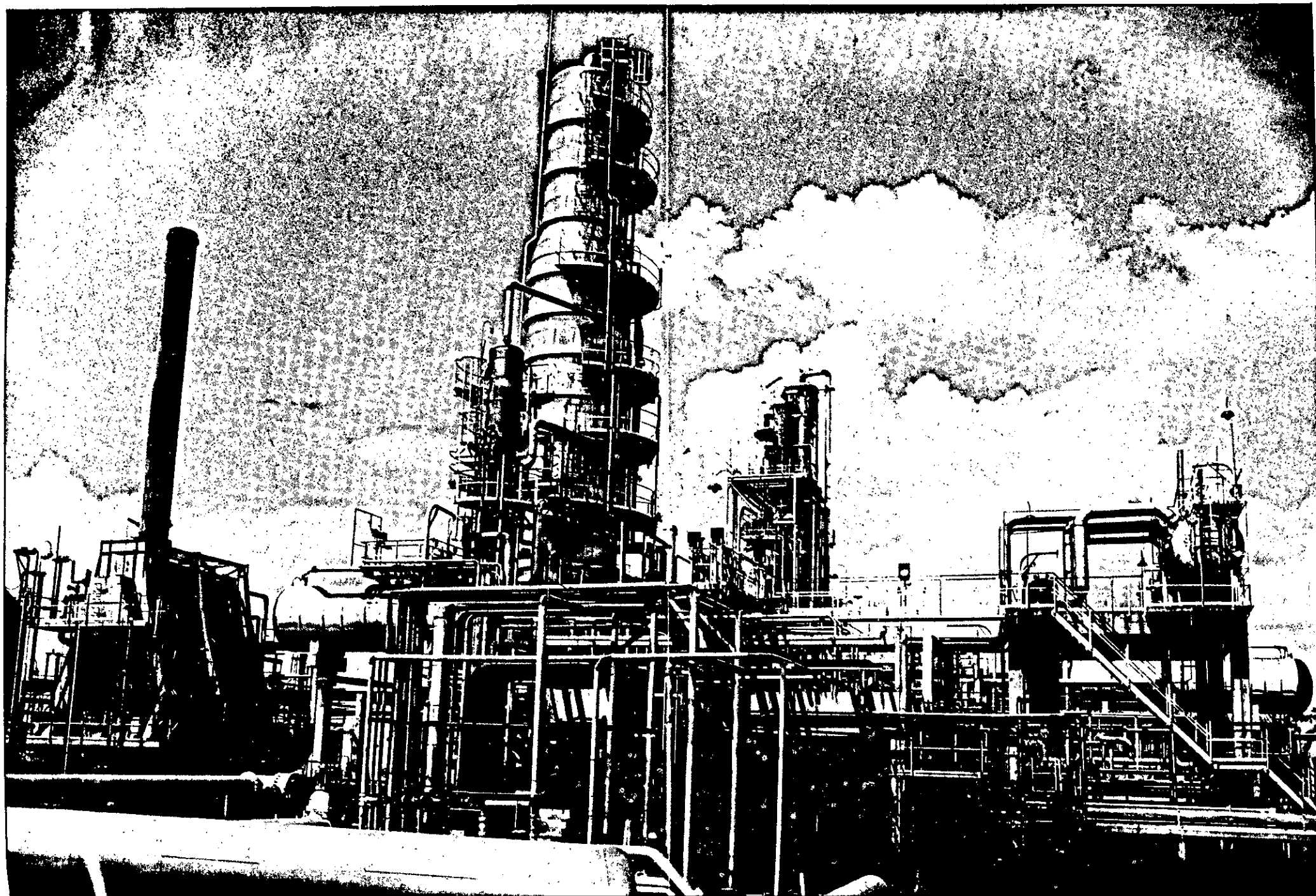
Refinaria Landulpho Alves - Unidade de Destilação a Vácuo do Sistema Lubrificante.
